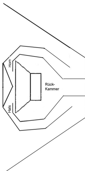
4. Zweiwegumlenkkompression
