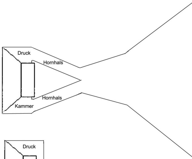
2. Zweiwegkompression
